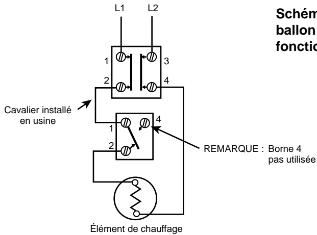
Circuit à un seul élément avec débranchement complet des deux fils d'alimentation
